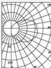
18W QUAD COMPACTO FLUORESCENTE
